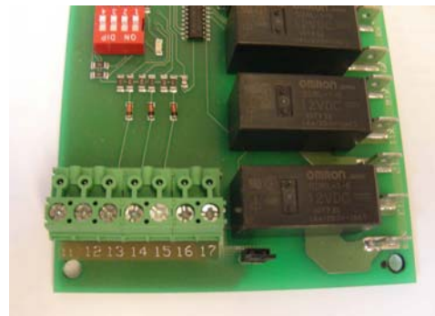
Маркировка соединительных зажимов схемной платы паровой установки HNS Touch
